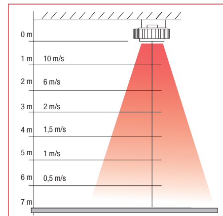
Luchtstroom
