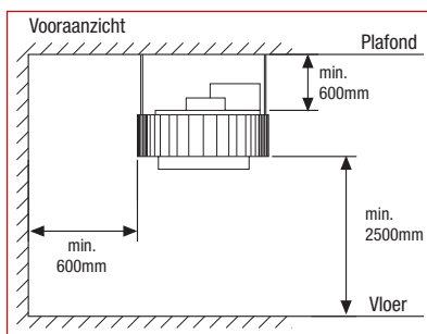
Veiligheidsafstanden (mm)
