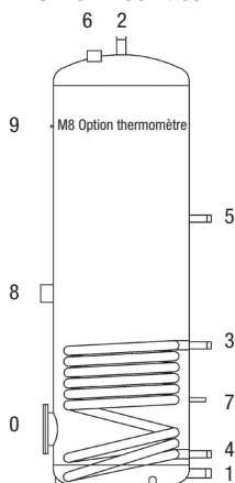
7 Doigt de gant pour sonde solaire
