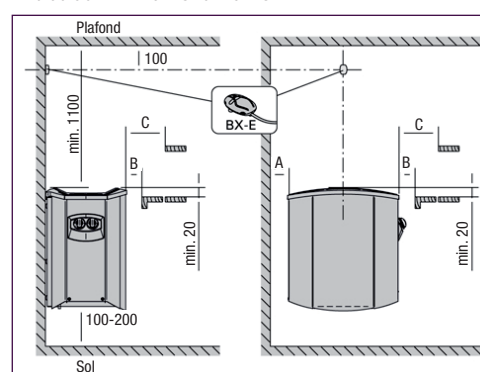
Dimensions en mm VEGA LUX &amp; VEGA LUX E
