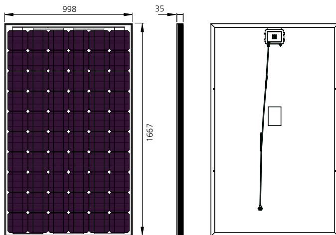
Premium L mono black Poids : 24 kg
