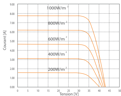
Données de référence pour le modèle HIT-H250E01 (Température des cellules: 25°C)
