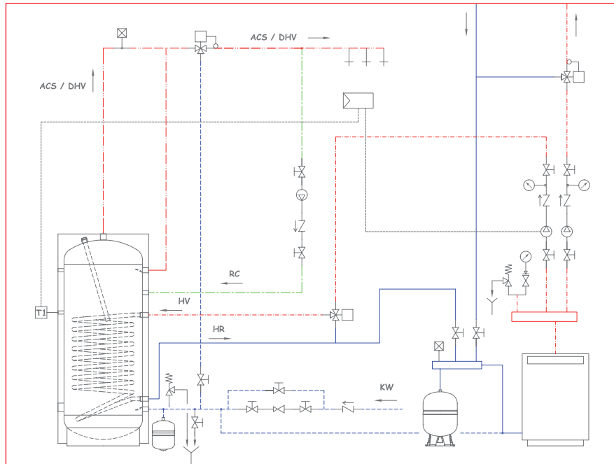
Schéma de principe vase d'expansion sanitaire et chauffage
